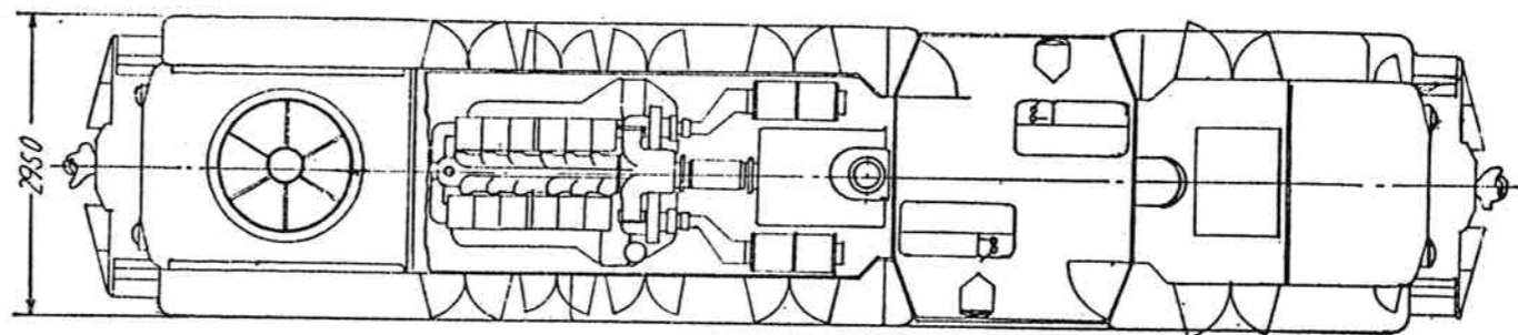
第1-5図 DE10形機関車形式図
